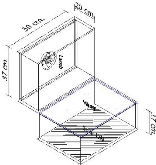
รูปที่ 1 เครื่องวัดความโปร่งแสงยางแผ่นผึ่งแห้ง
