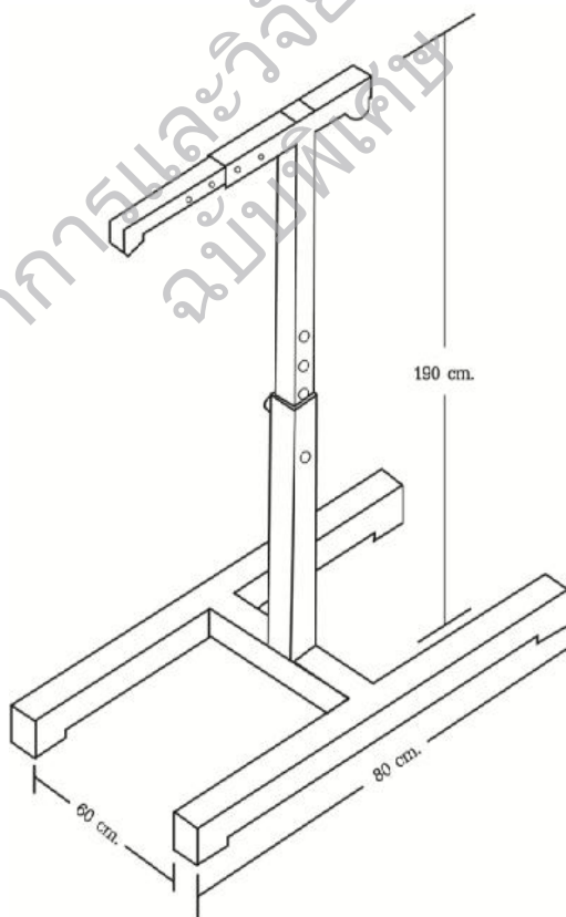
รูปที่ 2 ออกแบบโครงสร้างของเครื่องกายภาพบำบัดโรคหมอนรองกระดูกสันหลัง
