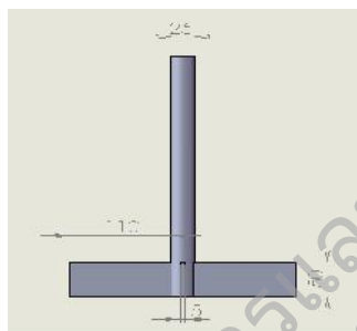
(ก) ใบกวนที่ออกแบบ
