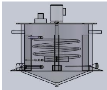
(ก) ลายเส้นถึงปฏิกรณ์
