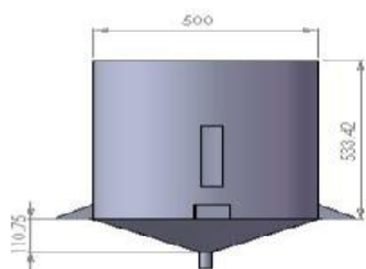
(ก) ลายเส้นถังล้างและแยกไขมัน
