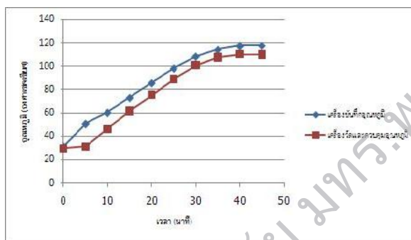
รูปที่ 7 การเพิ่มอุณหภูมิของน้ำมันสบู่ดำด้วยเครื่องวัดอุณหภูมิ 2 แบบ
