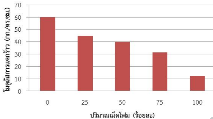
รูปที่ 11 โมดูลัสการแตกร้าวที่อายุ 28 วัน ของแผ่นเฟอร์โรซีเมนต์
