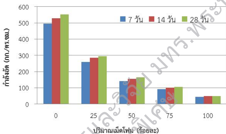
รูปที่ 7 กำลังอัดของคอนกรีต
