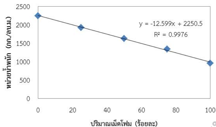
รูปที่ 9 ความสัมพันธ์ระหว่างหน่วยน้ำหนักที่อายุ 28 วันกับปริมาณเมล็ดโพม
