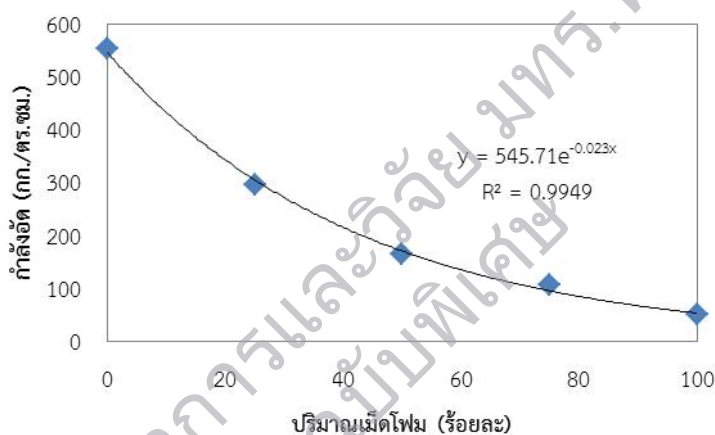
รูปที่ 10 ความสัมพันธ์ระหว่างกำลังอัดที่อายุ 28 วันกับปริมาณเมล็ดโพม
