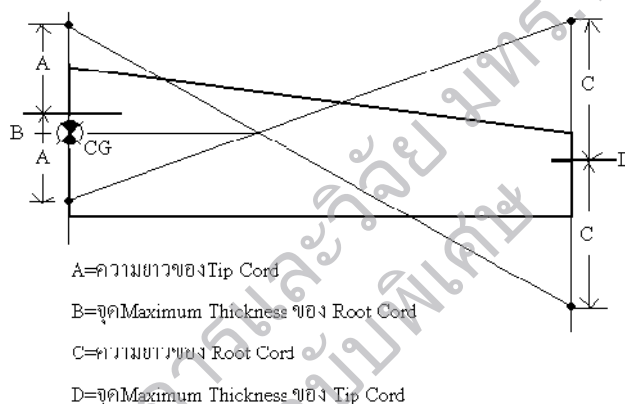
รูปที่ 2 การหาดำแหน่งของ Center of gravity (CG)
