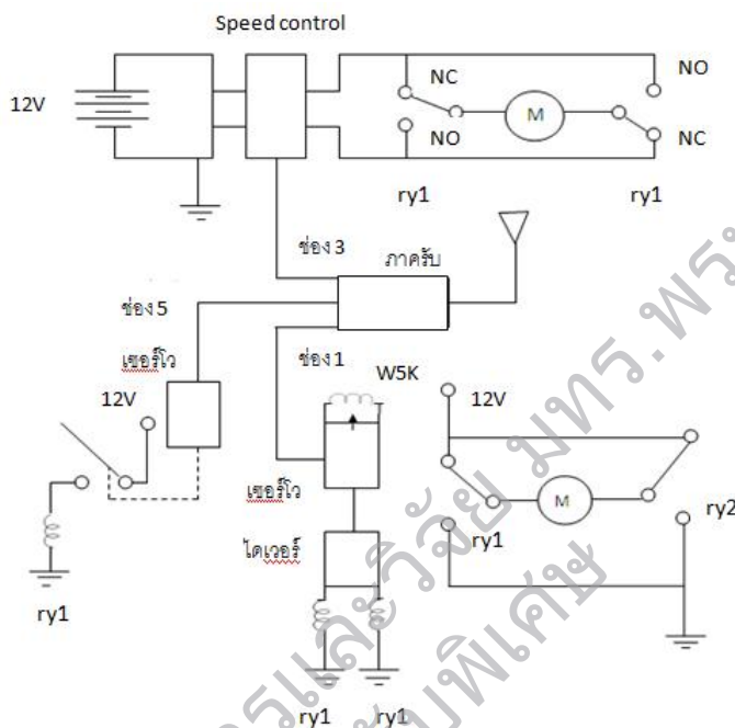
รูปที่ 4 หลักการทำงานของวงจรควบคุม (Mungme N, Duangmane W, Loday A, 2010.)
