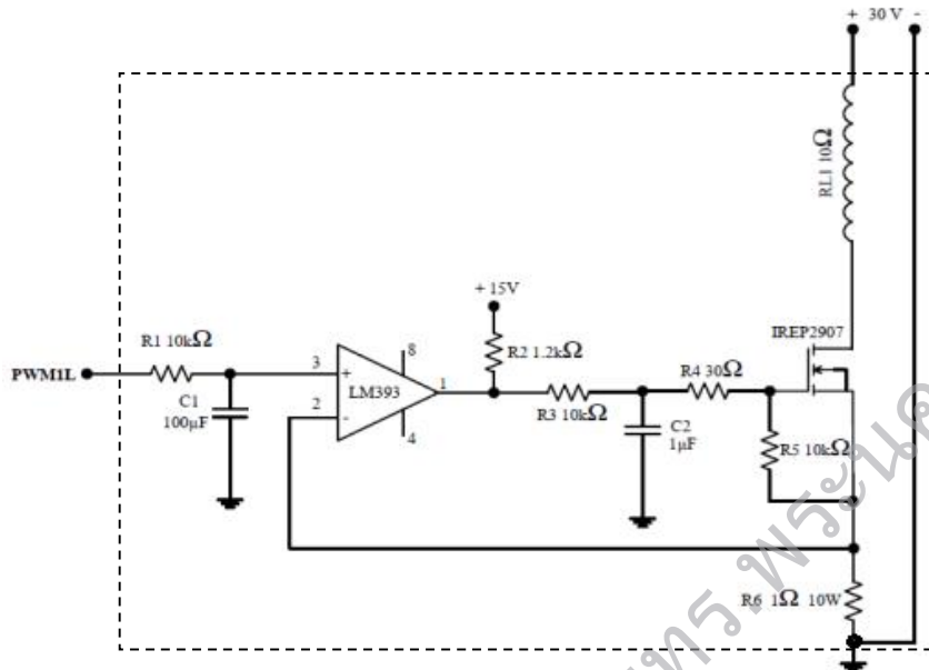
รูปที่ 2 วงจรภาคกำลังของอิเล็กทรอนิกส์ไหลดที่เสนอ
