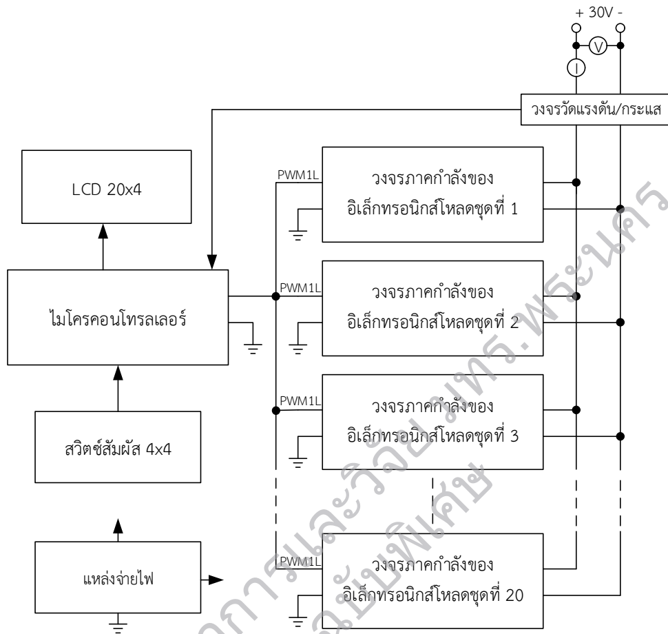
รูปที่ 3 ไดอะแกรมระบบโดยรวมของอิเล็กทรอนิกส์โหลดที่เสนอ
