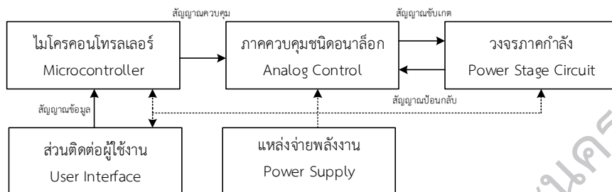
รูปที่ 1 ไดอะแกรมของระบบอิเล็กทรอนิกส์ไหลตที่เสนอ
