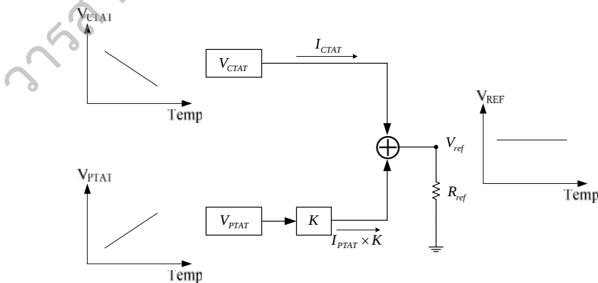
รูปที่ 1 บล็อกไดอะแกรมวงจรอ้างอิงแรงดันแบบซีมอส
