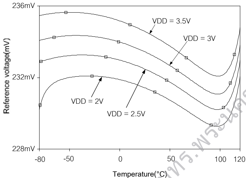
รูปที่ 5 แรงดันอ้างอิงเมื่ออุณหภูมิที่มีแหล่งจ่ายแรงดัน 2V, 2.5V, 3V และ 3.5V
