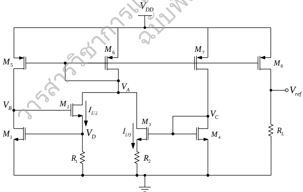
รูปที่ 2 วงจรอ้างอิงแรงดันแบบซีมอสที่น่าเสนอ
