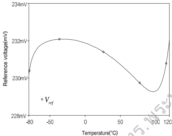
รูปที่ 3 แรงดันอ้างอิงเมื่อมีการเปลี่ยนแปลงอุณหภูมิ
