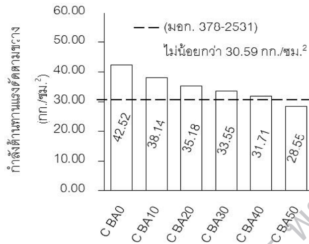
รูปที่ 4 กําลังต้านทานแรงดัดตามขวางของแผ่นคอนกรีตปูนซีเมนต์ประเภทที่ 1 ล้วน และปูนซีเมนต์แทนที่ด้วยเถ้าขานอ้อย
