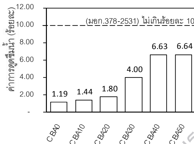
รูปที่ 3 การดูดซึมน้ำของตัวอย่างแผ่นคอนกรีตปูนซีเมนต์ประเภทที่ 1 ล้วน และปูนซีเมนต์แทนที่ด้วยเถ้าขาน้อย
