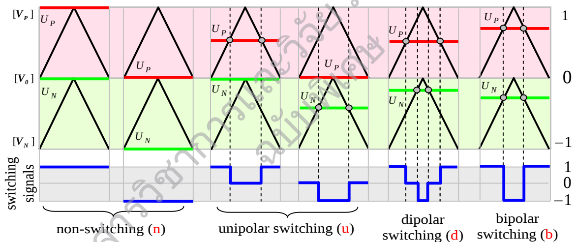
รูปที่ 3 การมอดูเลตโดยอาศัยคลื่นพาหะแบบซัฟฟ์ของอินเวอร์เตอร์ 3 ระดับ
