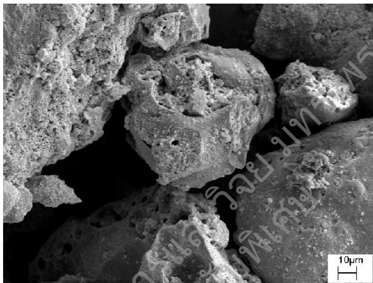
รูปที่ 2 ภาพกำลังขยายสูง (SEM) ของเถ้าก้นเตา (350X)
