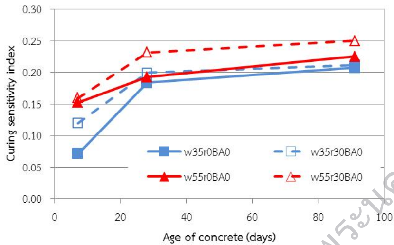
รูปที่ 8 เปรียบเทียบค่า CSI ที่อายุ 28 วัน ของคอนกรีตที่ผสมและไม่ผสมเถ้าลอย
