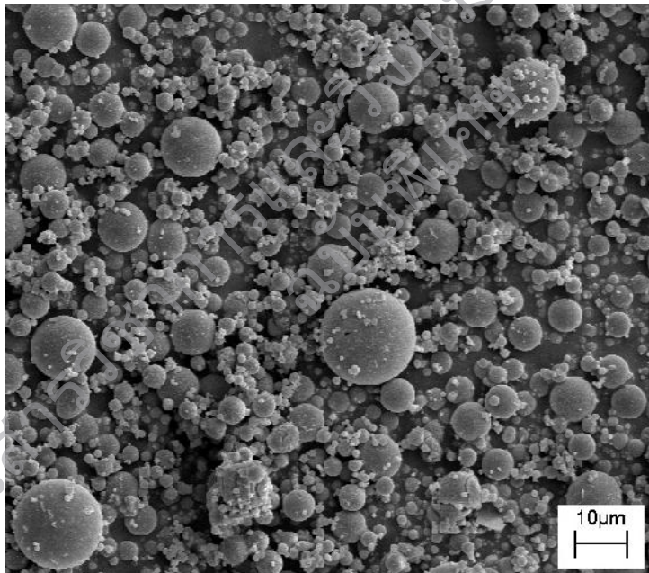
รูปที่ 1 ภาพกล้องจุลทรรศน์ของเถ้าลอย (500X)
