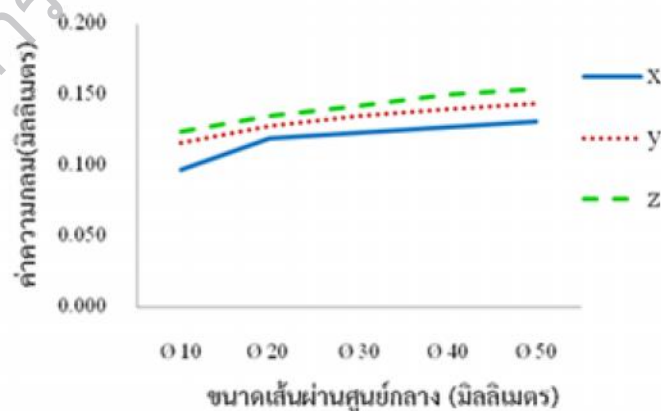
รูปที่ 8 แสดงแนวโน้มค่าความคลาดเคลื่อนความกลมเฉลี่ยของชิ้นงานขนาดเส้นผ่านศูนย์กลาง 10 20 30 40 และ 50 มิลลิเมตร
