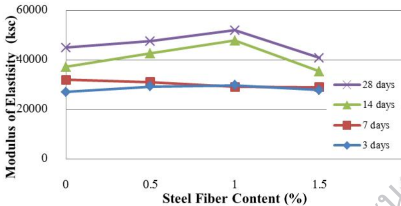
รูปที่ 10 ความสัมพันธ์ระหว่าง Modulus of Elasticity กับ Steel Fiber Content (%)
