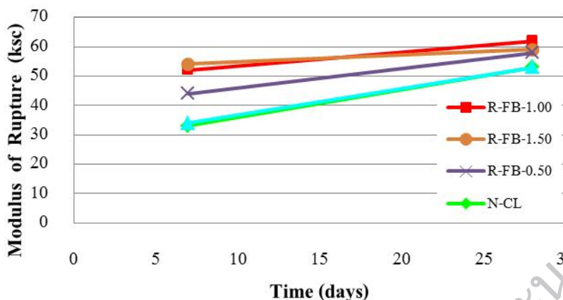
รูปที่ 8 ความสัมพันธ์ระหว่างกำลังดัดของคอนกรีตกับอายุการบ่มต่างๆ
