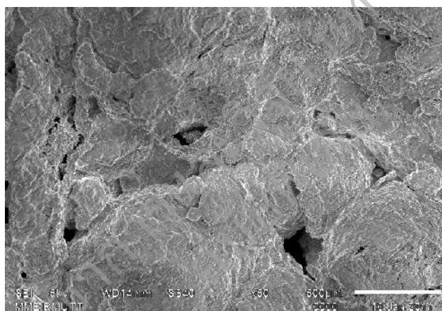
รูปที่ 4 คอนกรีตบล็อกดินขาวผสมเส้นใยกากมะพร้าว ด้วยกล้อง SEM กำลังขยาย 50 เท่า
