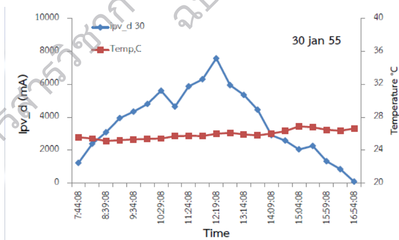
รูปที่ 10 แสดงการเปรียบเทียบค่ากระแส lpv\_d กับค่าอุณหภูมิ วันที่ 30 มกราคม 2555
