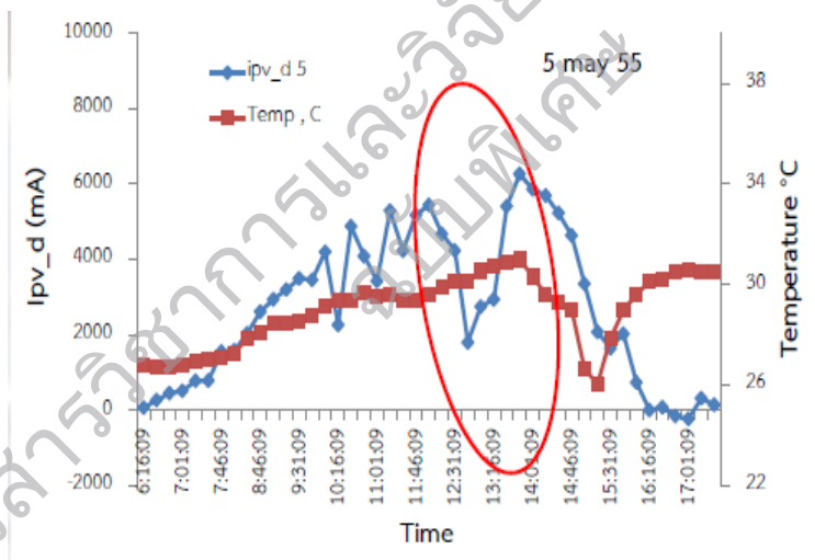
รูปที่ 4 แสดงการเปรียบเทียบค่ากระแส Ipv_d กับค่าอุณหภูมิ วันที่ 5 พฤษภาคม 2555
