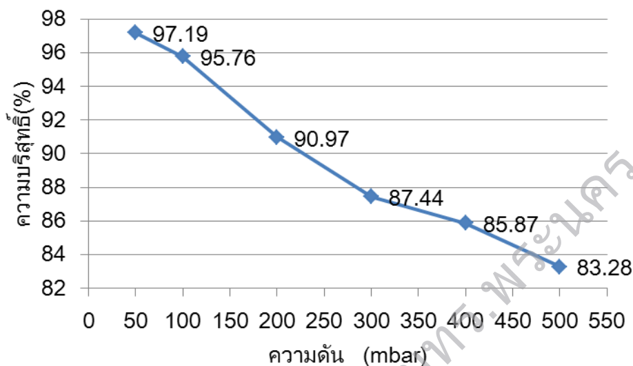
รูปที่ 1 ร้อยละความบริสุทธิ์ของสารละลาย N-Methyl-Pyrrolidone ภายใต้สภาวะความดันความดัน 50 – 500 mbar
