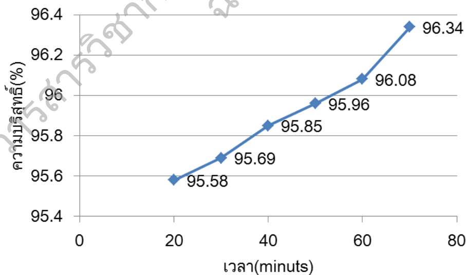
รูปที่ 2 แสดงเปอร์เซ็นต์ความบริสุทธิ์ของสารละลาย N-Methyl-Pyrrolidone ที่เวลา 20 – 70 นาที
