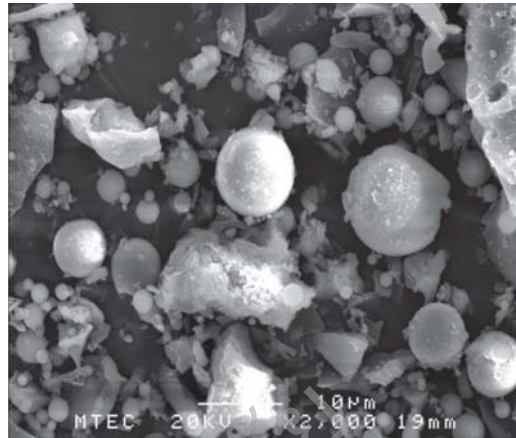
รูปที่ 1 ลักษณะอนุภาคของเถ้าแกลบผสมเถ้าลอย
