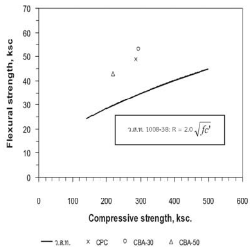
รูปที่ 2 ความสัมพันธ์ระหว่างกำลังดัดกับกำลังอัดของคอนกรีตผสมเถ้าแกลบร่วมกับเถ้าลอย
