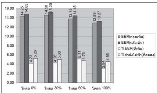
รูปที่ 9 ผลการทดสอบที่อุณหภูมิรอบตัวควบแน่น 50 องศาเซลเซียส
