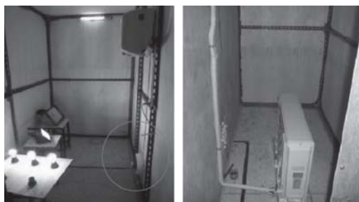
a) ห้องปรับอากาศ b) ห้องควบแน่น
