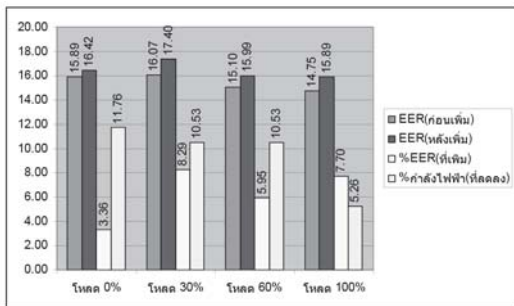
รูปที่ 8 ผลการทดสอบที่อุณหภูมิโดยรอบชุดเครื่องควบแน่น 40 องศาเซลเซียส
