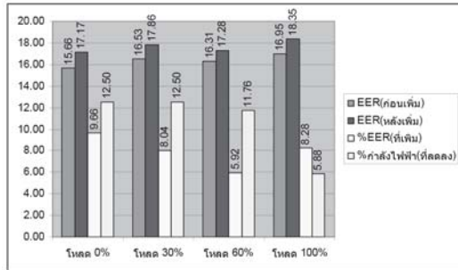
รูปที่ 7 ผลการทดสอบที่อุณหภูมิรอบตัวควบแน่น 30 องศาเซลเซียส
