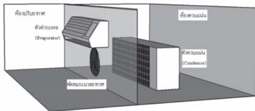
รูปที่ 2 โครงสร้างห้องทดสอบการเพิ่มประสิทธิภาพ เครื่องปรับอากาศโดยใช้ลมจากพัฒลมระบายอากาศ
