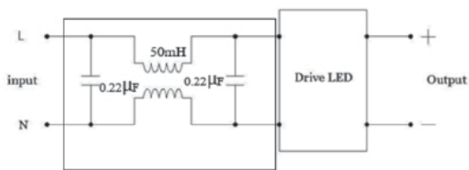
รูปที่ 12 วงจรลดสัญญาณรบกวนคลื่นแม่เหล็กไฟฟ้า
