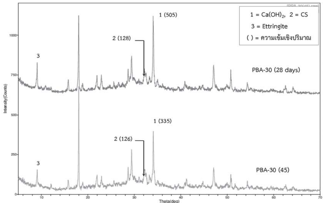
รูปที่ 6 ปริมาณสารประกอบของซีเมนต์เฟสท์ PBA-30 ที่อายุ 28 วัน เปรียบเทียบกับ PBA-30(45)
