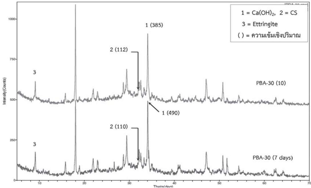
รูปที่ 5 ปริมาณสารประกอบของซีเมนต์เฟสท์ PBA-30 ที่อายุ 7 วัน เปรียบเทียบกับ PBA-30(10)
