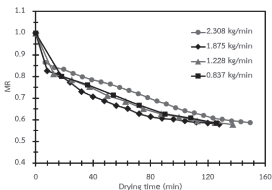
รูปที่ 3 กราฟแสดงความสัมพันธ์ระหว่างอัตราส่วนความชื้นกับเวลาที่ใช้อบแห้งที่อัตราการไหลข้าวเปลือกต่างกัน
