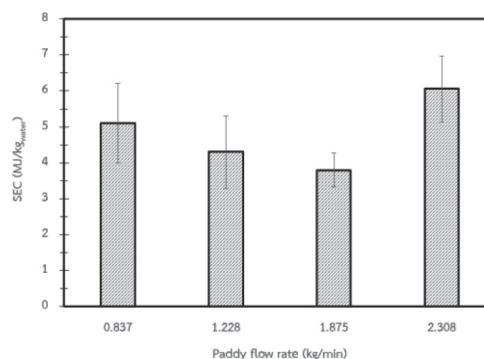
รูปที่ 5 ค่าความสิ้นเปลืองพลังงานจำเพาะของการอบแห้งข้าวเปลือกที่อัตราการไหลข้าวเปลือกต่างกัน
